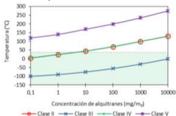
Fig 1. Punto de rocío de las clases de alquitranes 2-5, en función de la temperatura y concentración. Fuente: Tomado y adaptado de [8]
